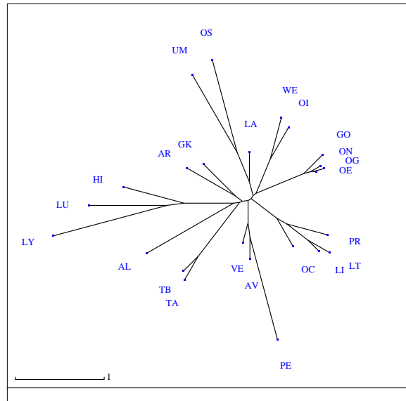
(b) LT_{NJ}
