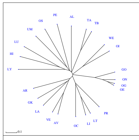
(f) T_{UPGMA}
